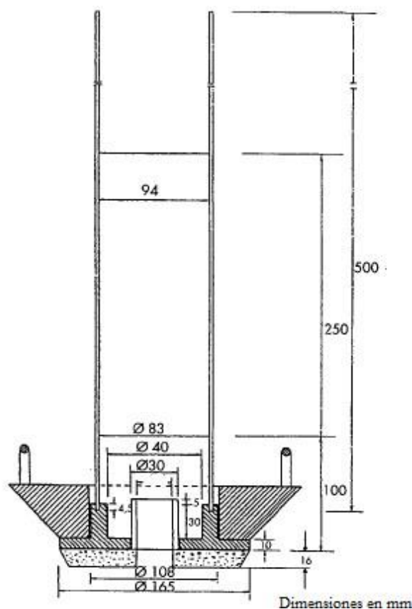
Figura 796 - 1. Permeámetro LCS
